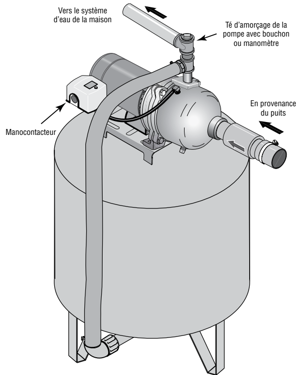
Figure 2 : Branchements sur un réservoir préchargé
